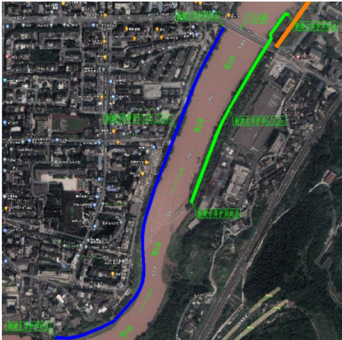
图 1.1-2 新建望鱼镇三台段左岸护岸起止位置图
